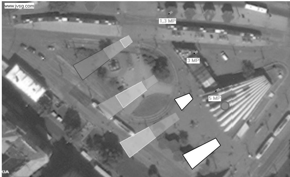
7. ábra Arcfelismerési zónák 60 méter referenciatáv esetén
